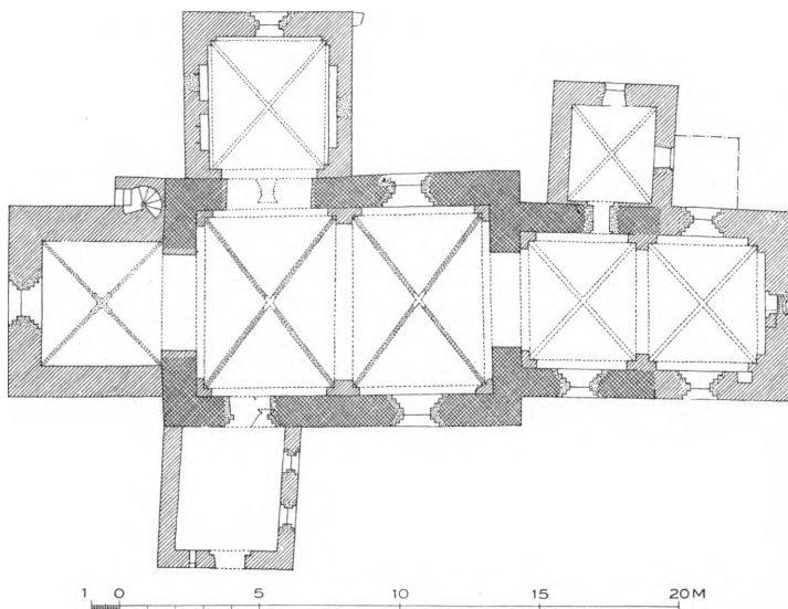
Fig. 2. Beldringe. Plan. 1:300. Maalt af Th. Havning 1915 (Arne Nystrøm 1929).
